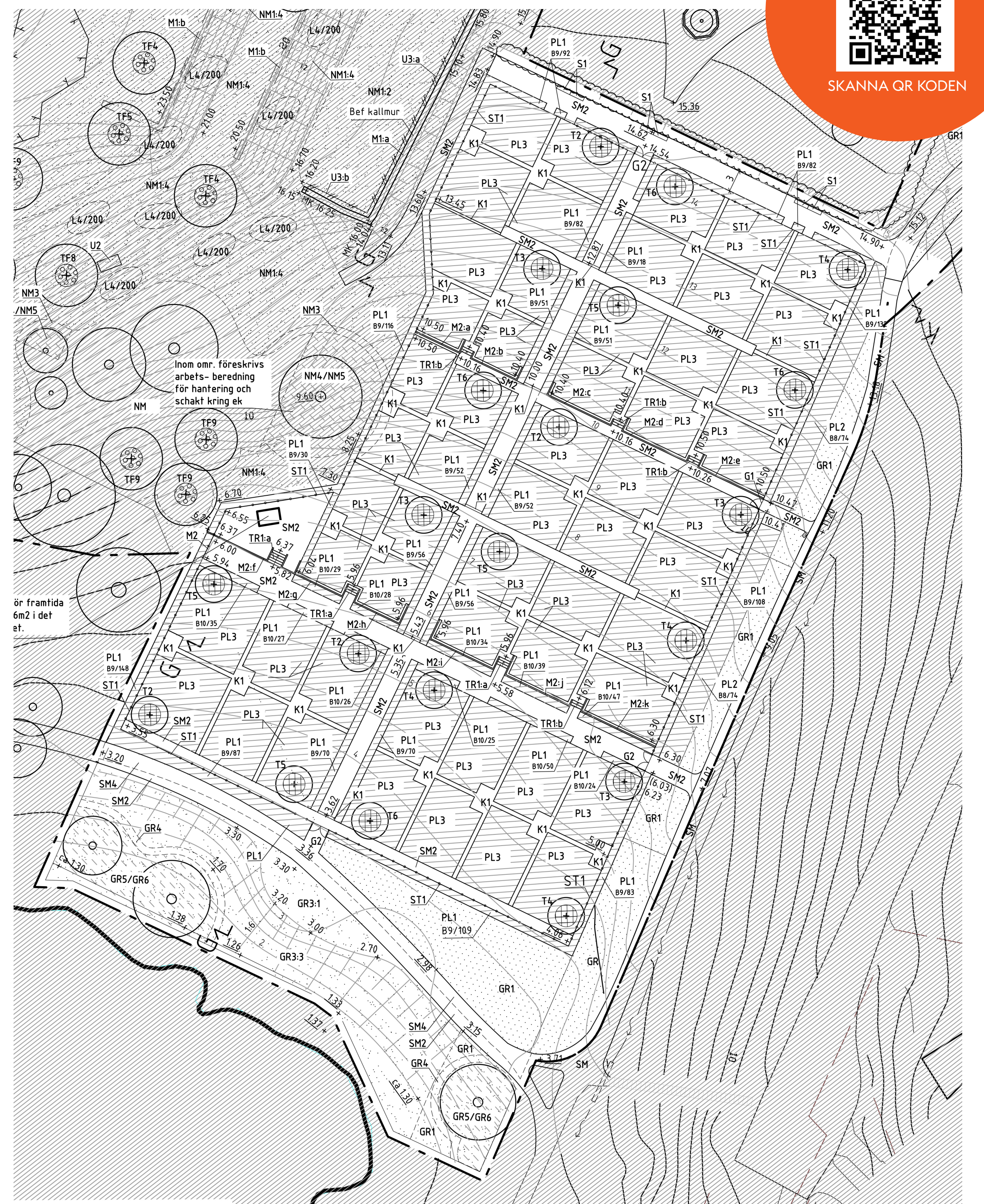
Ritning över Koloniområdet.
